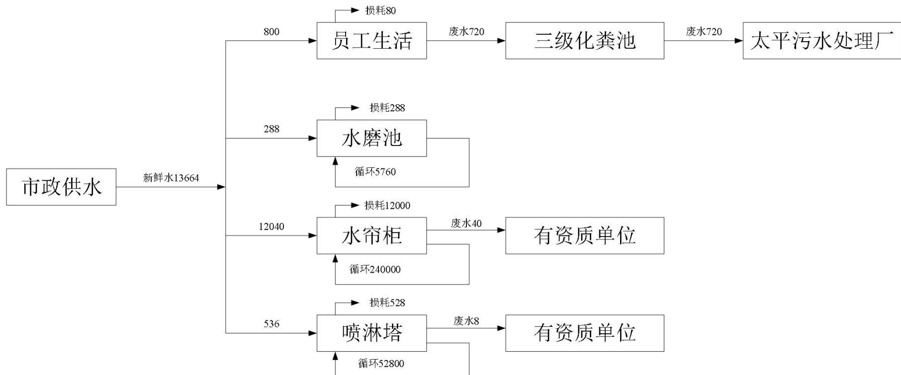
图 2-1 本项目水平衡图 单位: m³/a
