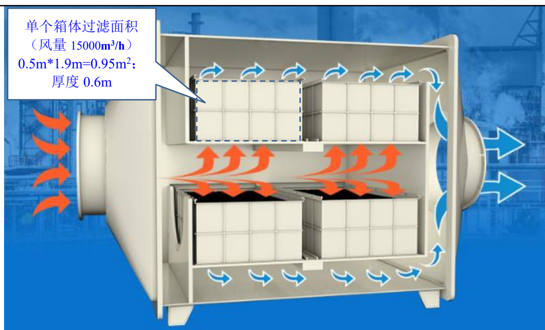
图4-2活性炭箱内部结构及风走向图
