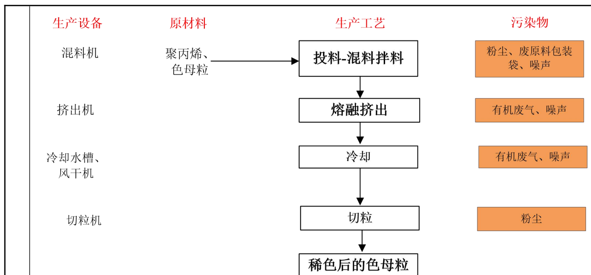
图 2-4 色母稀色生产工艺流程及产污环节
