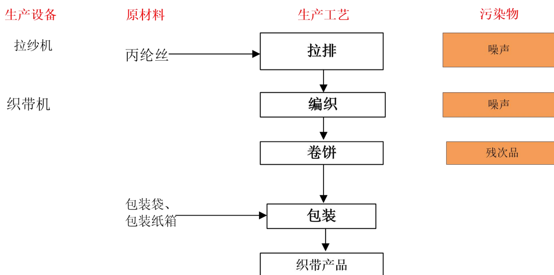
图 2-3 项目织带产品生产工艺流程图
