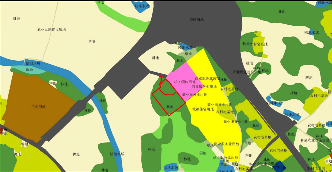
落实前《清远市国土空间总体规划（2021-2035）》土地使用规划图局部
