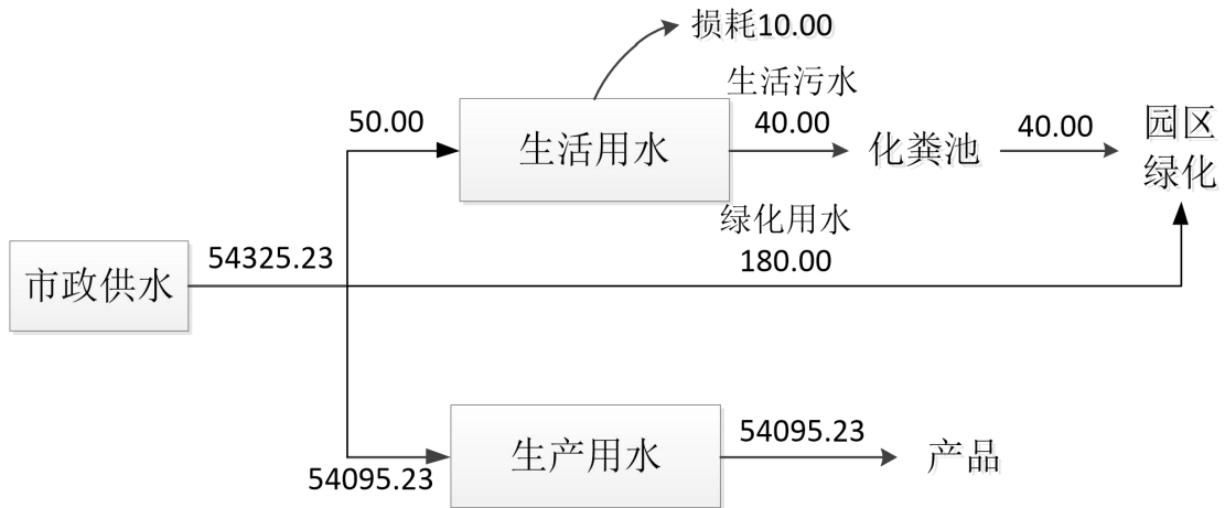
图 2-4 扩建后项目水平衡图（单位：t/a）
