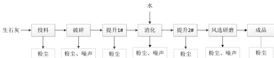
图 2-4 氢氧化钙生产工艺流程图
