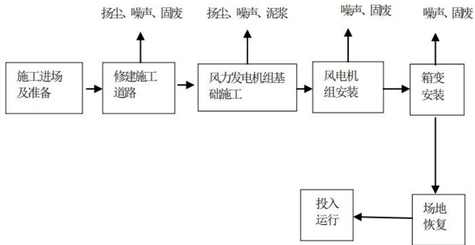
图 2-1 风电场施工工艺流程图
