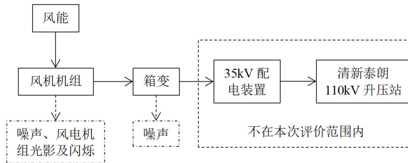
图 2-5 运营期工艺流程图
