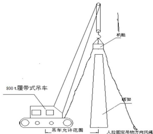
图 2-3 机舱吊装示意图
