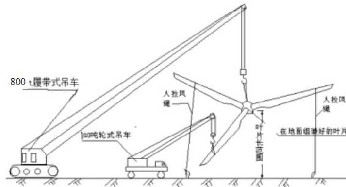
图 2-4 叶片吊装示意图
