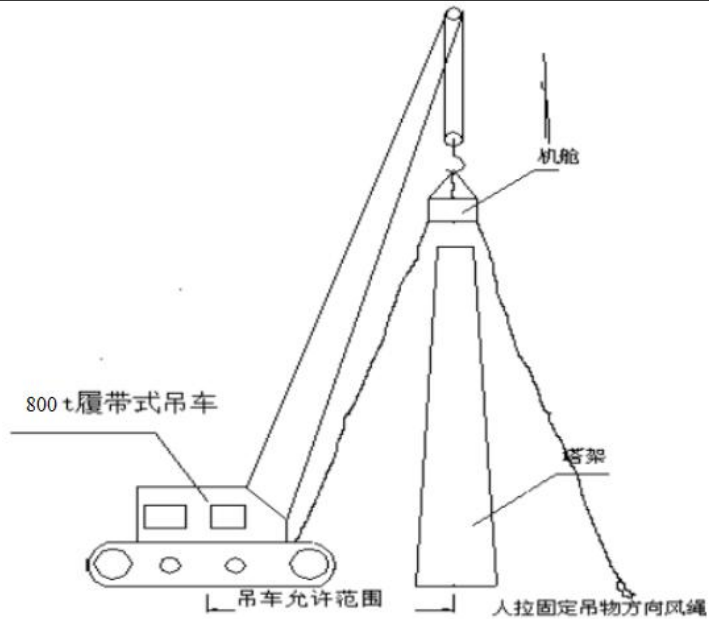
图 2-3 机舱吊装示意图
