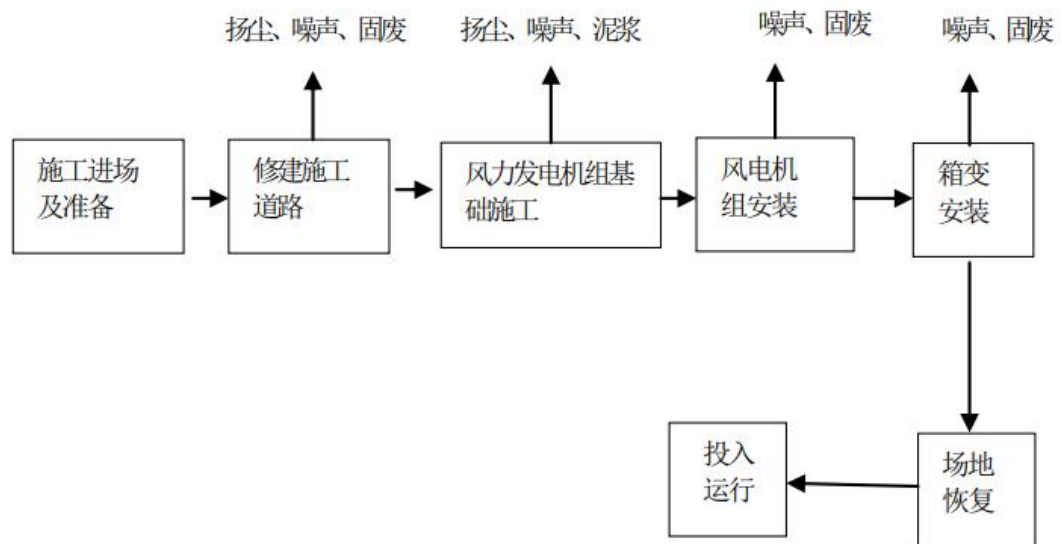
图 2-1 风电场施工工艺流程图
