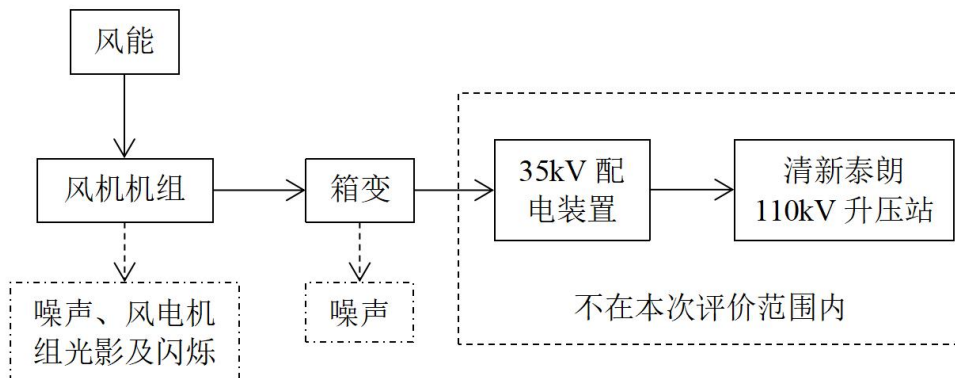
图 2-5 运营期工艺流程图
