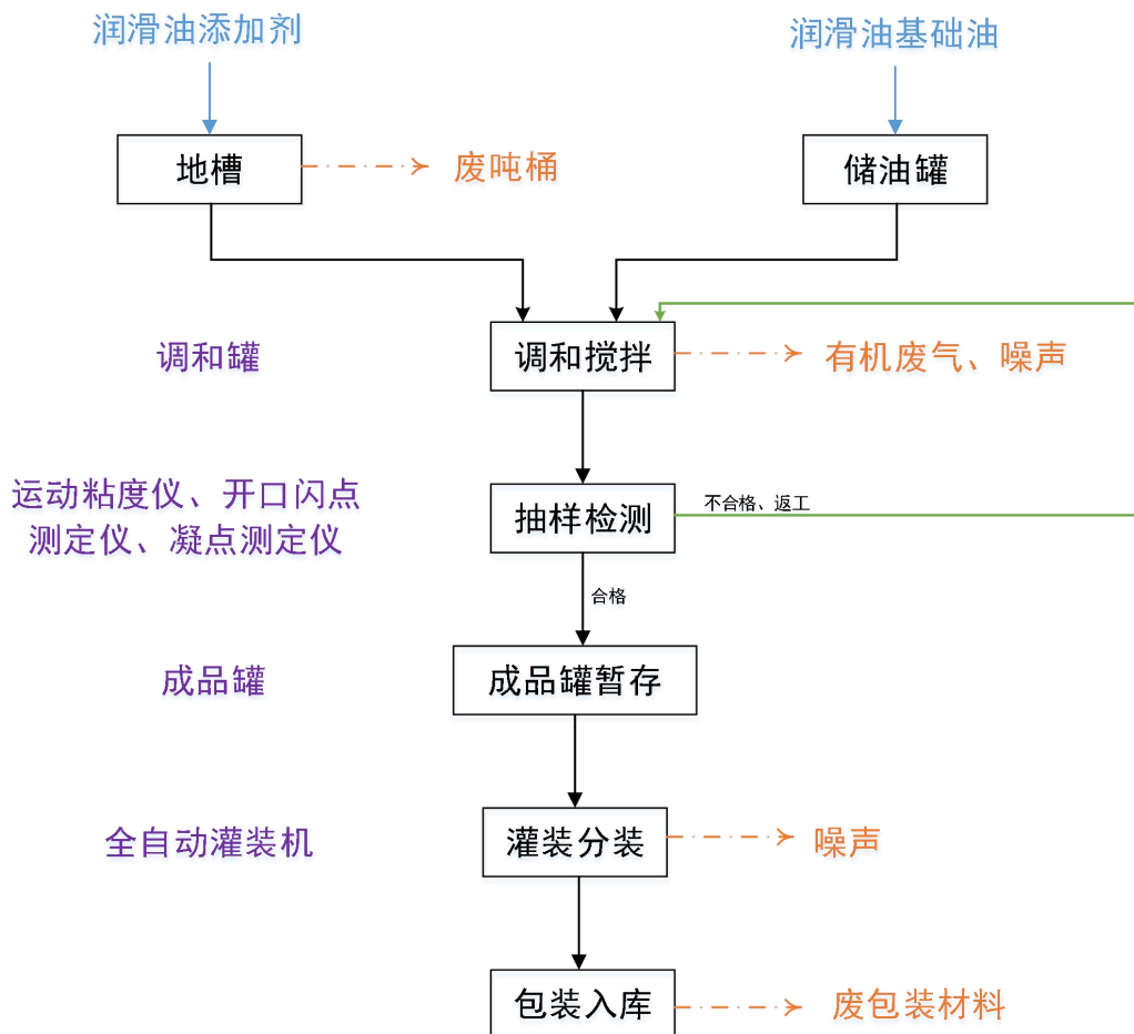
图 2-2 项目润滑油产品生产工艺流程图
