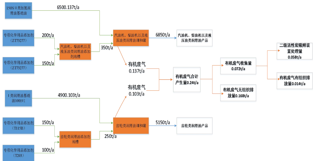
图 2-1 本项目物料平衡图
