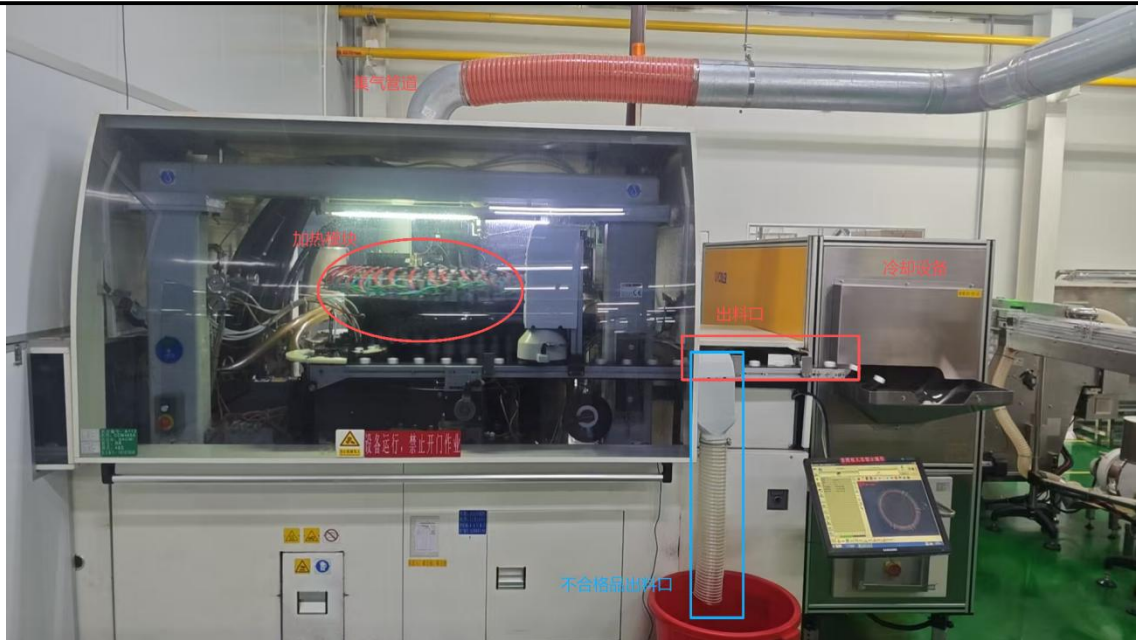
图 4-1 现有项目塑盖成型设备密闭情况图片
