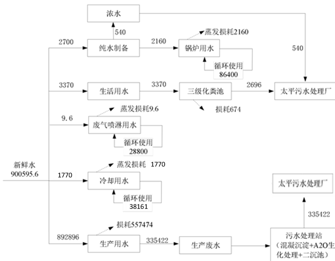
图 2-2 扩建后全厂水平衡图 m³/a
