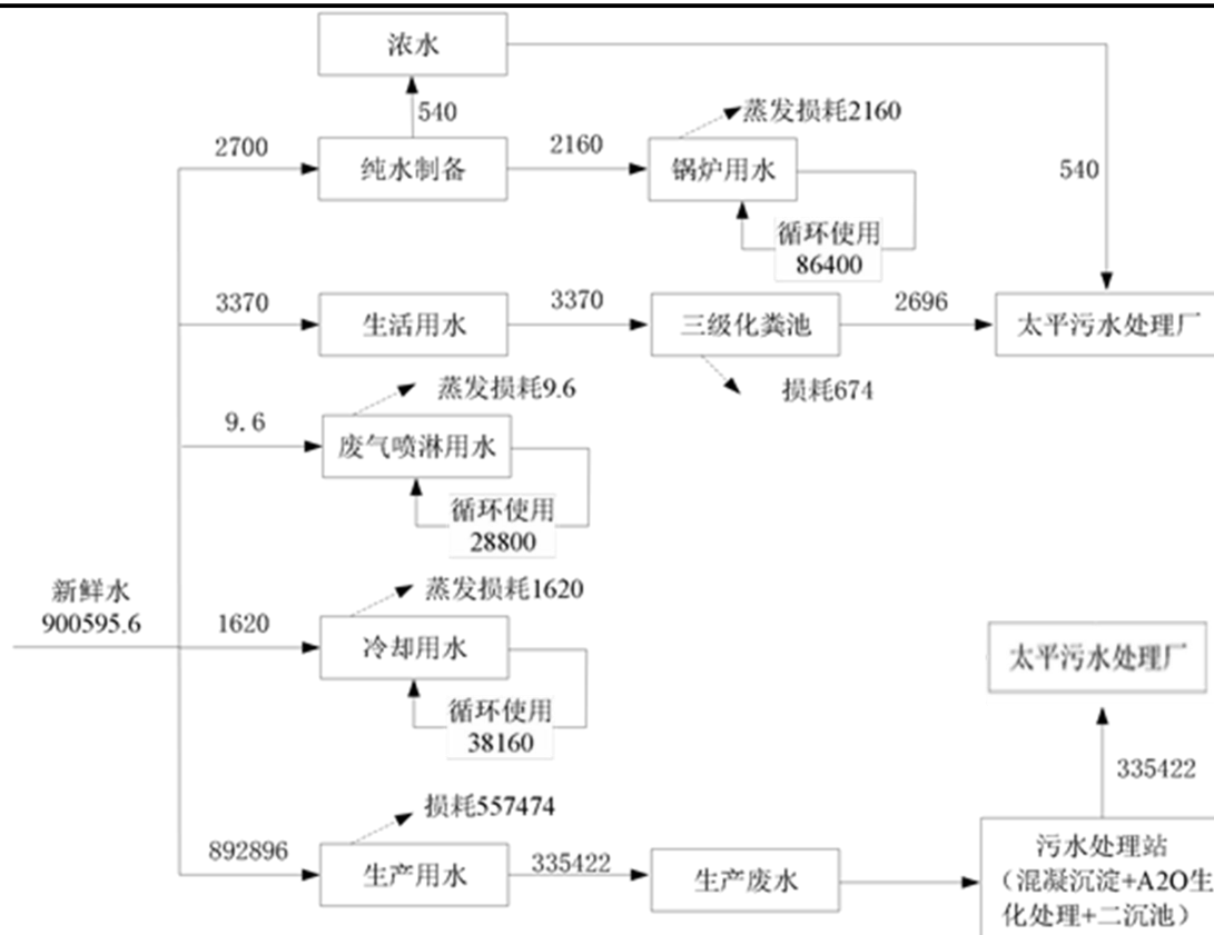
图 2-1 扩建前项目水平衡图 m³/a
