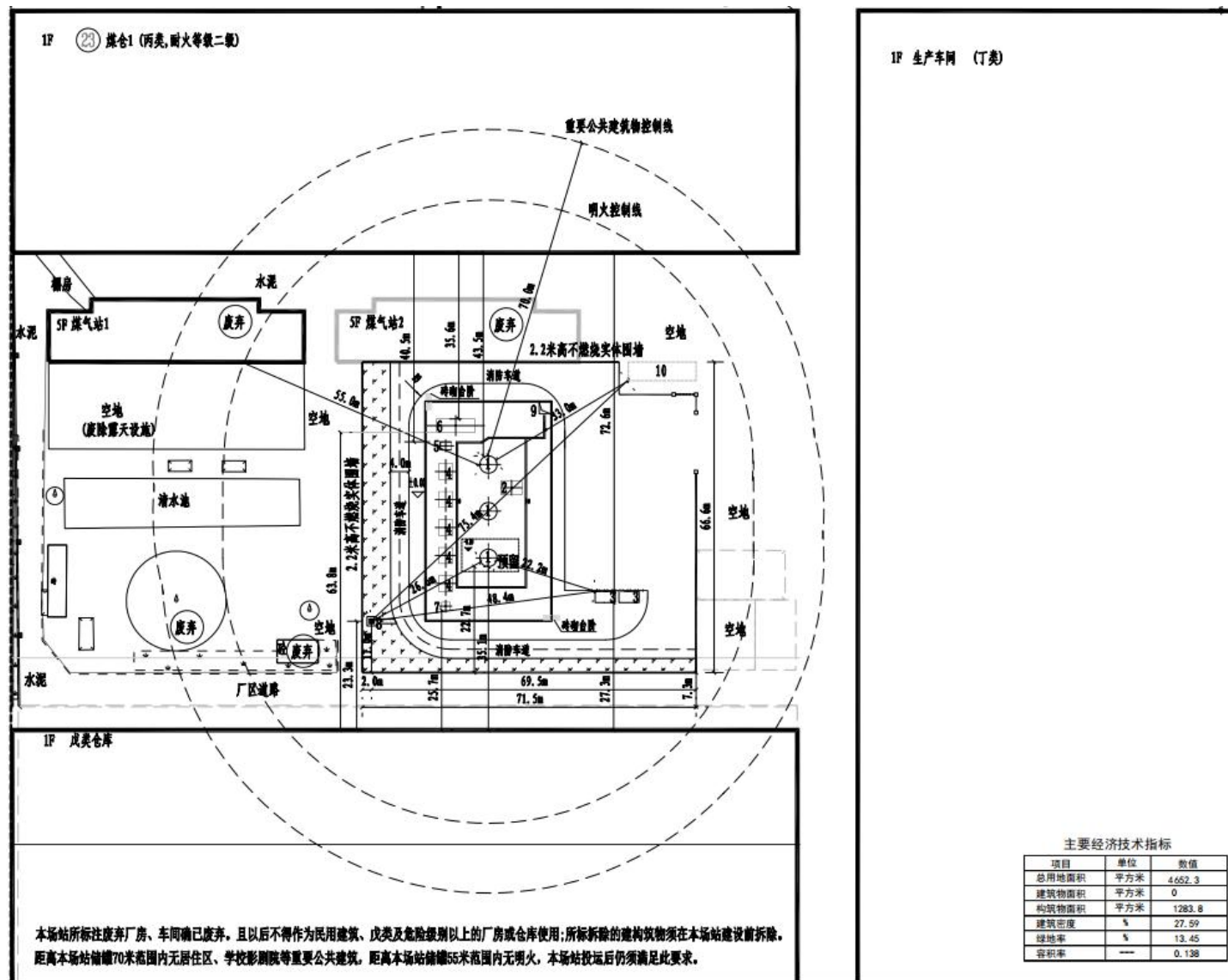
附图 6 项目平面布置图
